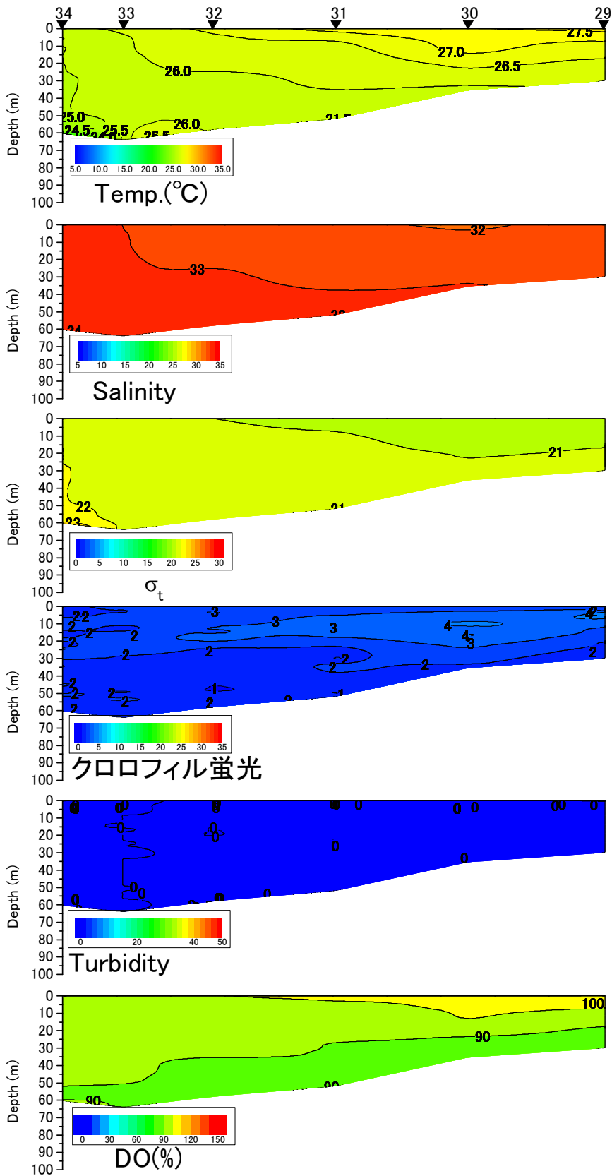
八代海西ラインの水温(°C)、塩分、密度( \sigma_t )、クロロフィル蛍光強度、濁度、溶存酸素飽和度(DO%)の鉛直面図(国土交通省の調査による) (2016年8月25日)
